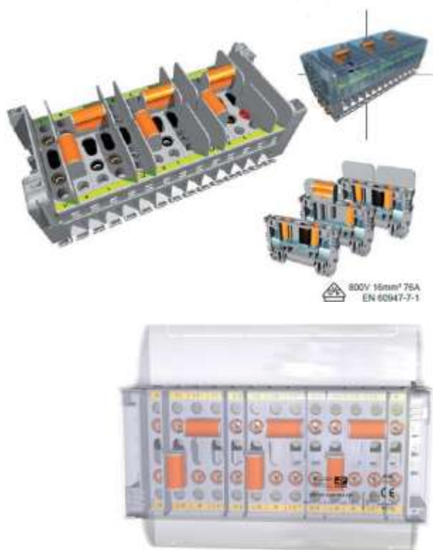
Svorkovnice ViD 13E 4t-9i CB EPI
