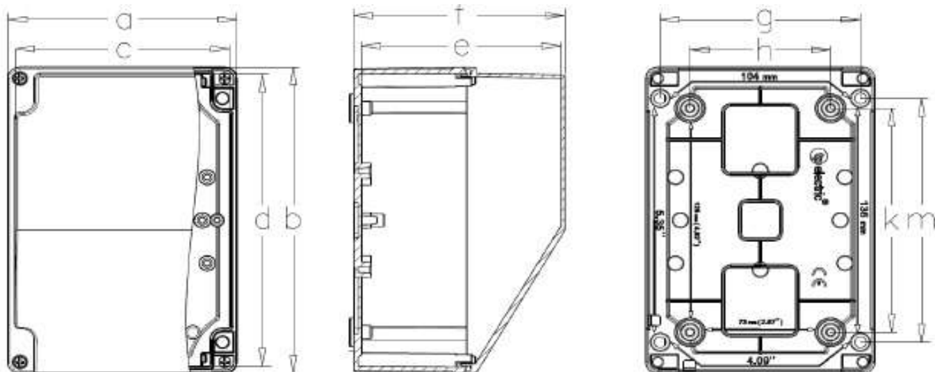
Rozměry boxu 3317 IP67
