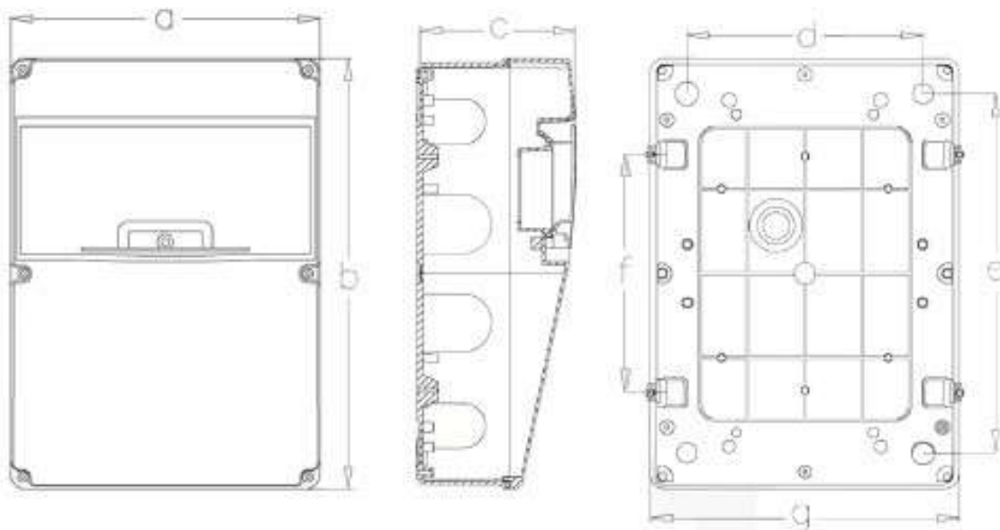
Rozměry boxu 3519 IP66
